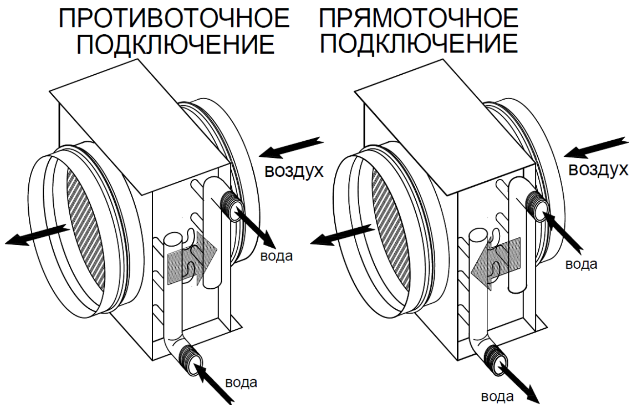
Рисунок 5.1 – Прямоточное и противоточное подключение
