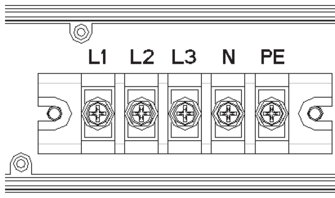
11 кВт/22 кВт трехфазный пятипроводной
