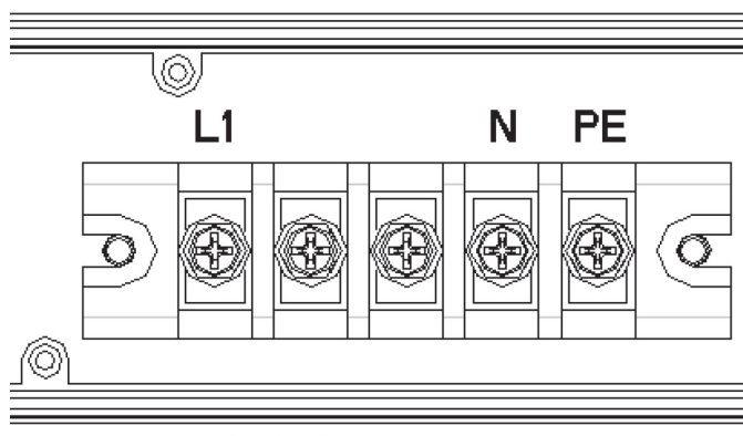
7 кВт однофазный трехпроводной
