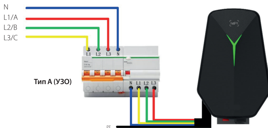
Чертеж автоматического выключателя за пределами зарядного устройства для электромобилей переменного тока 11 кВт/22 кВт
