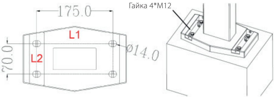
Схема 7.2.2 Параметры установочных отверстий для основания зарядной станции (единица измерения: мм)
