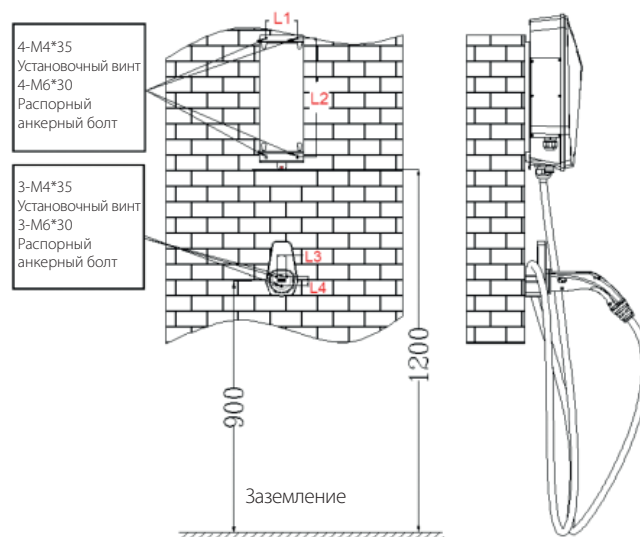
Параметр установочных отверстий дополнительной опоры (единица измерения: мм)
